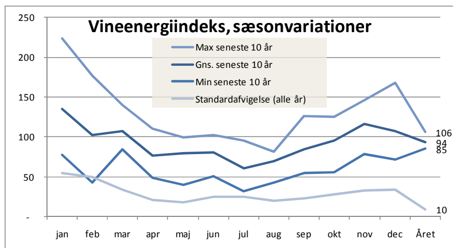
Figur 51: Sæsonmæssig variation i vindressourcen. Labels yderst til højre viser årsværdier, seneste 10 år er således 6% under langtidforventning. Standardafvigelsen på årsværdien er 10%
