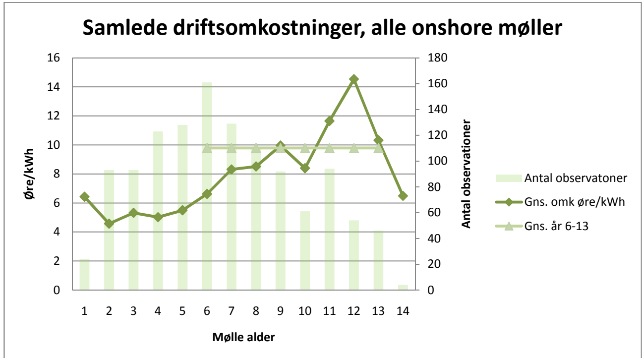
Figur 5 Samtlige vindmøller >= 600 kW med driftsdataoplysninger. År 6-13 vurderes at repræsentere levetidsomkostningen bedst, idet perioden er efter diverse garantiordninger.
