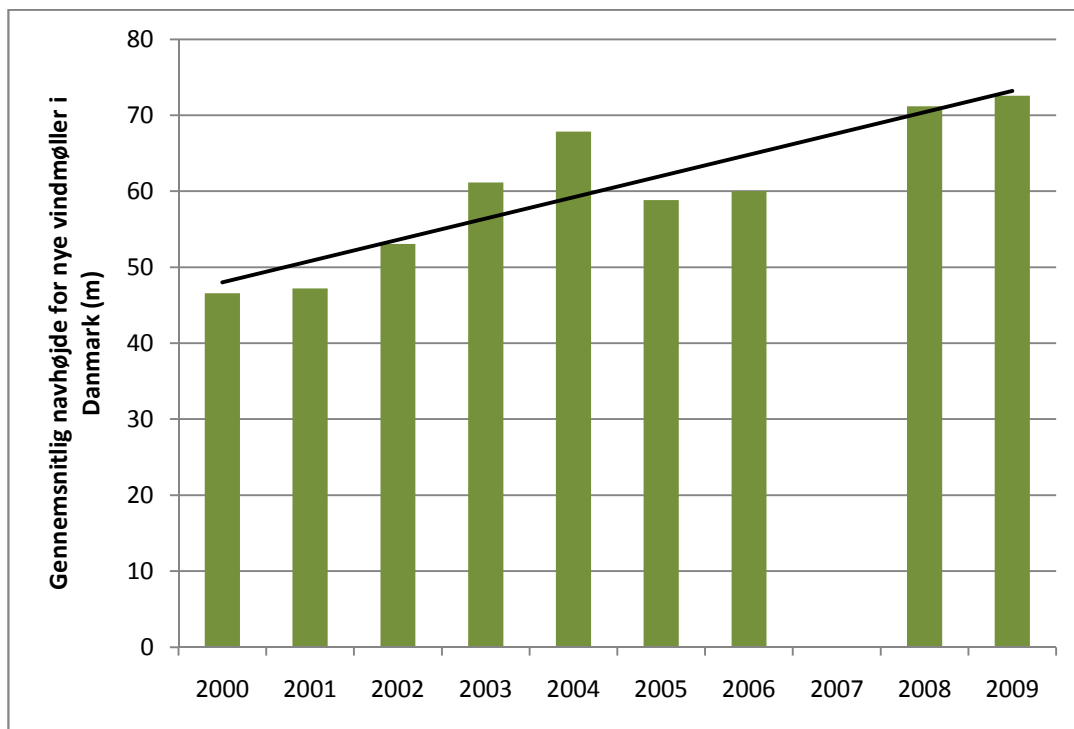
Figur 37 Årlige gennemsnitlige navhøjde for nye landbaserede vindmøller installeret i Danmark fra 2000 til 2009
