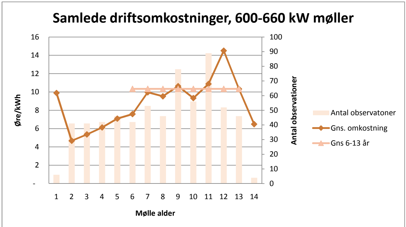
Figur 6 Den gruppe møller der er statistisk bedst repræsenteret er gruppen 600-660kW - denne har samtidig den længste track record af den nyere generation af vindmøller, der har en betydelig lang driftshistorie.
