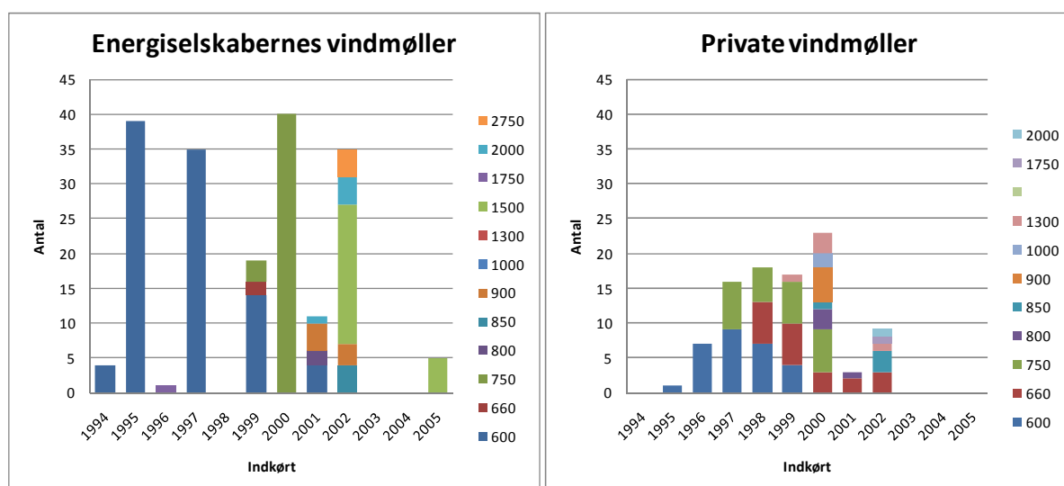
Figur 4 Vindmøllerne i driftsøkonomianalysen fordelt på indkøringsår og effekt for hhv. Energiselskabsejede og private. Energiselskabernes vindmøller er typisk opstillet i større parker.
