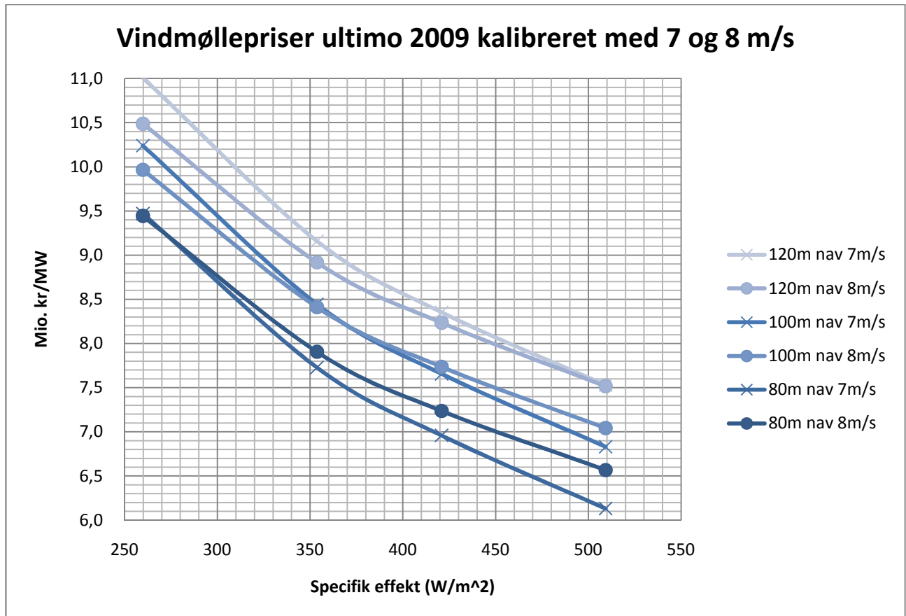
Figur 25 Hvis prisen beregneren i stedet kalibreres ved 7 m/s middelvind i 80 m højde, ville kurverne ændres lidt.
