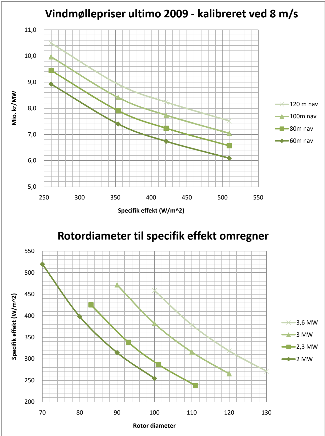
Figur 24 Med de to sæt grafer ovenfor er det relativt simpelt at gå ind at aflæse, hvad en given vindmølle ca. bør koste. Der er tale om vindmølle leveret, opstillet og indkørt i Danmark, men excl. fundament, eltilslutning mv. Der skal typisk tillægges 20%
